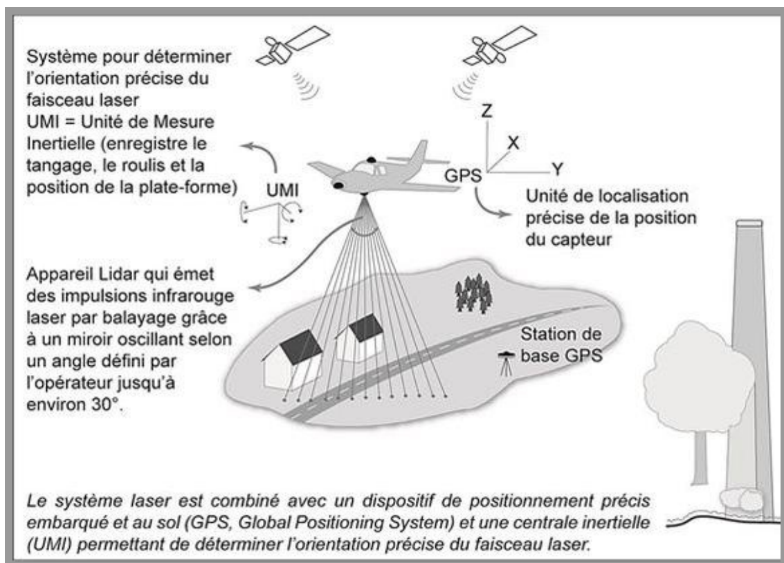
Principe du système laser aéroporté = LIDAR
